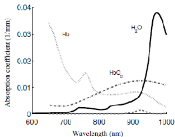
Figura 2 – Coeficientes de absorção para a água ( \text{H}_2\text{O} ), oxihemoglobina \text{HbO}_2 , desoxihemoglobina (Hb) e lipídios (abaixo), em escala – extraído de NISSILÄ et al, 2005 1 .
